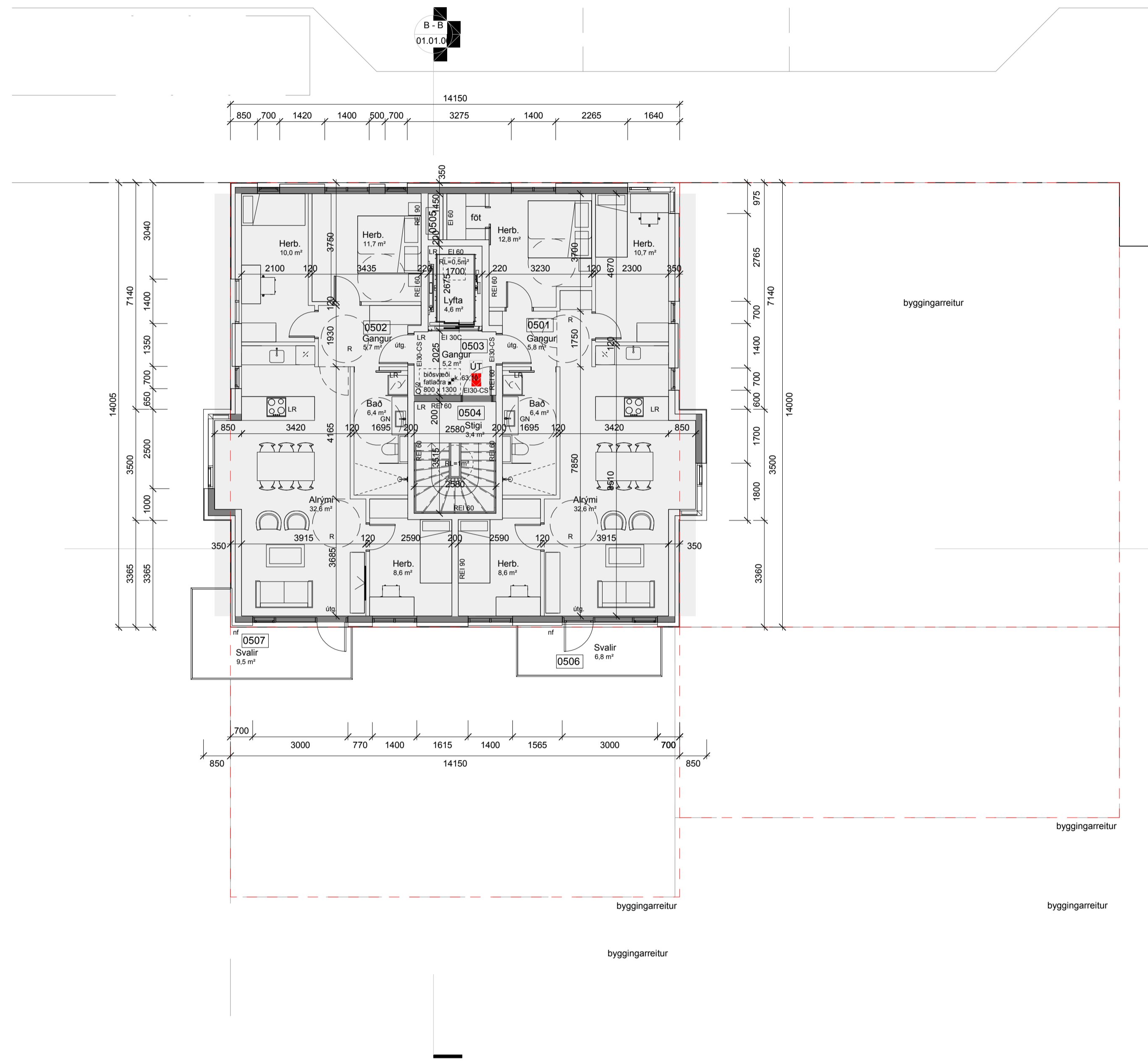
MHL 01_5. hæð 1:100
